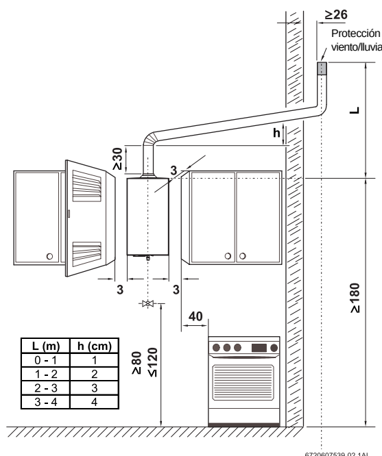
Fig. 4 Separaciones mínimas (en cm)
