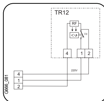
Fig. 7 - Conexión del regulador de temperatura. (Previamente eliminar puente entre 1 y 4, fig. 6, pos 163/1).
