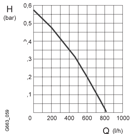
Diagrama del bomba
