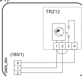
Fig. 8 - Conexión del regulador de temperatura. (Previamente eliminar puente entre 1 y 4, fig. 6, pos. 163/1)
