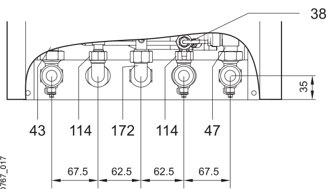
Placa de conexión sobre pared
