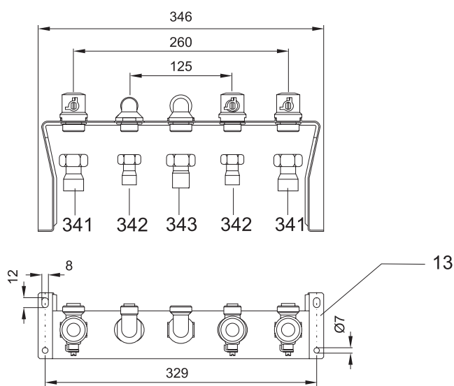
Placa de conexión
