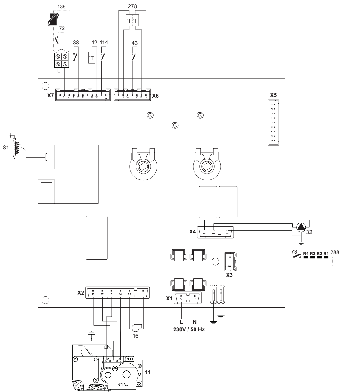
fig. 21 - Esquema eléctrico
