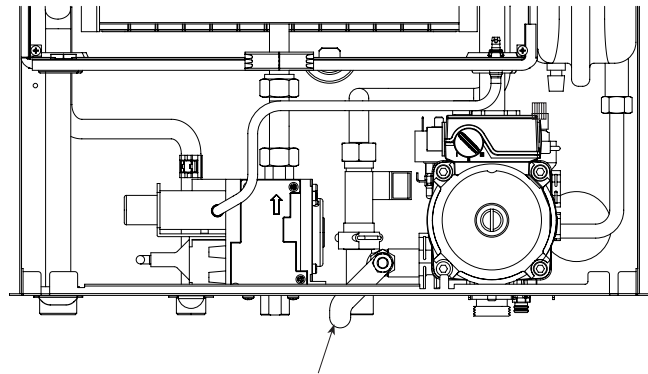
fig. 2 Llave de carga de la instalación
