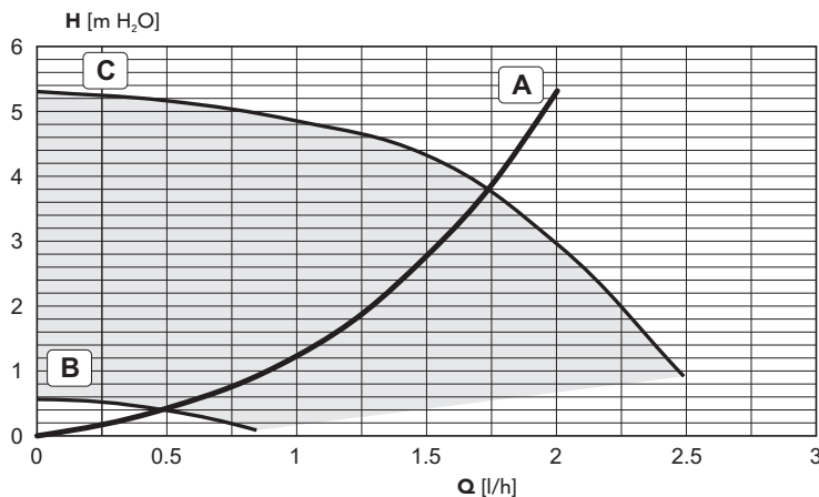
рис. 29 - Потеря напора/Напор циркуляционных насосов BLUEHELIX PRO 32 C
