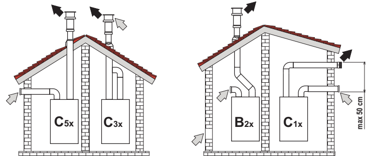
мал. 17 - Приклад підключення за допомогою відокремлених труб ( ⇨ = Повітря / ⇨ = Відпрацьовані газы )
