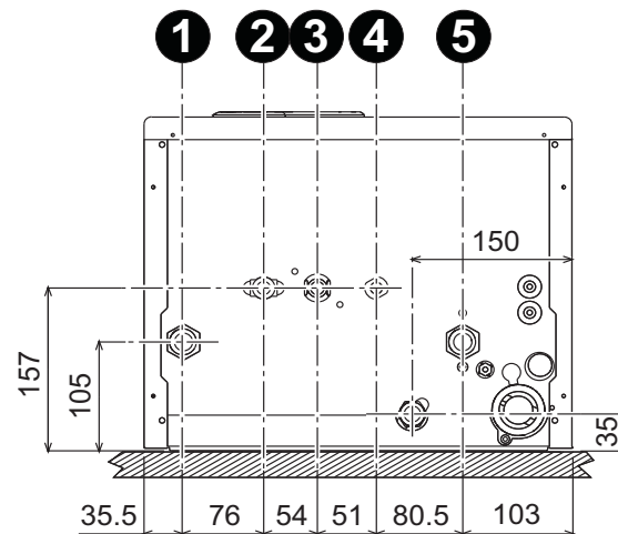
рис. 13 - Гидравлические штуцеры
