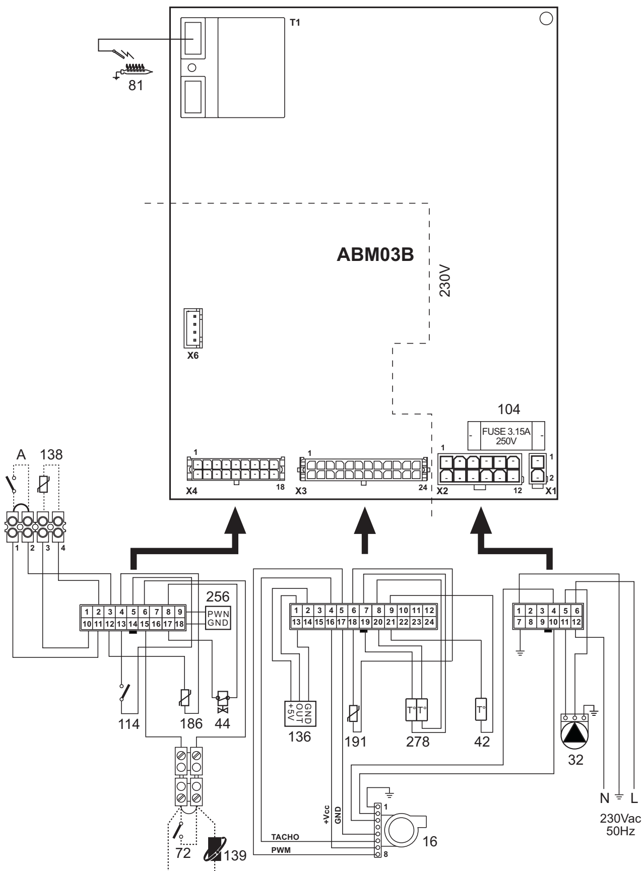
fig. 30 - Schema elettrico
