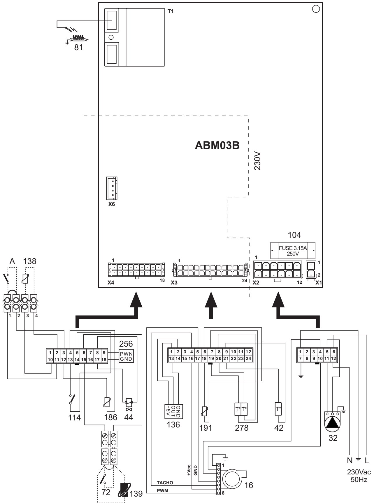
fig. 30 - Schéma électrique
