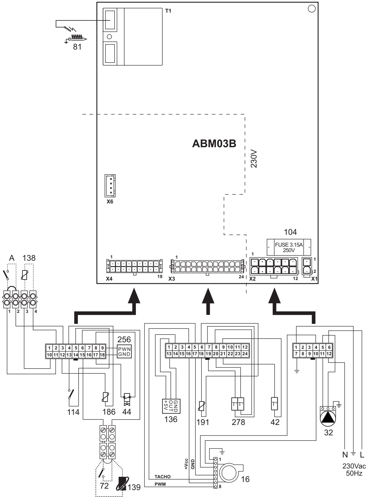
рис. 30 - Электрическая схема
