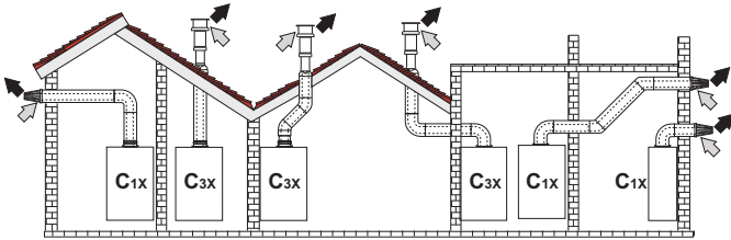
мал. 15 - Приклад підключення за допомогою співісних (коаксіальних) труб ( ⇨ = Повітря / ⇨ = Відпрацьовані газы )
