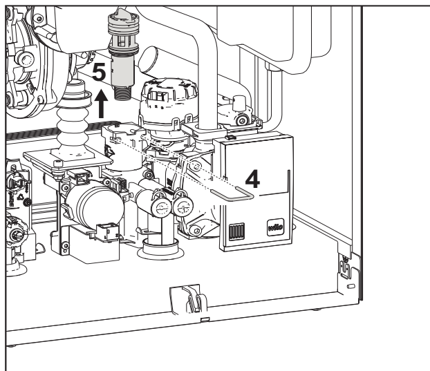
fig. 47- Caudalímetro
