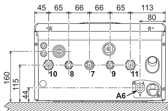
fig. 56- Vista inferior
