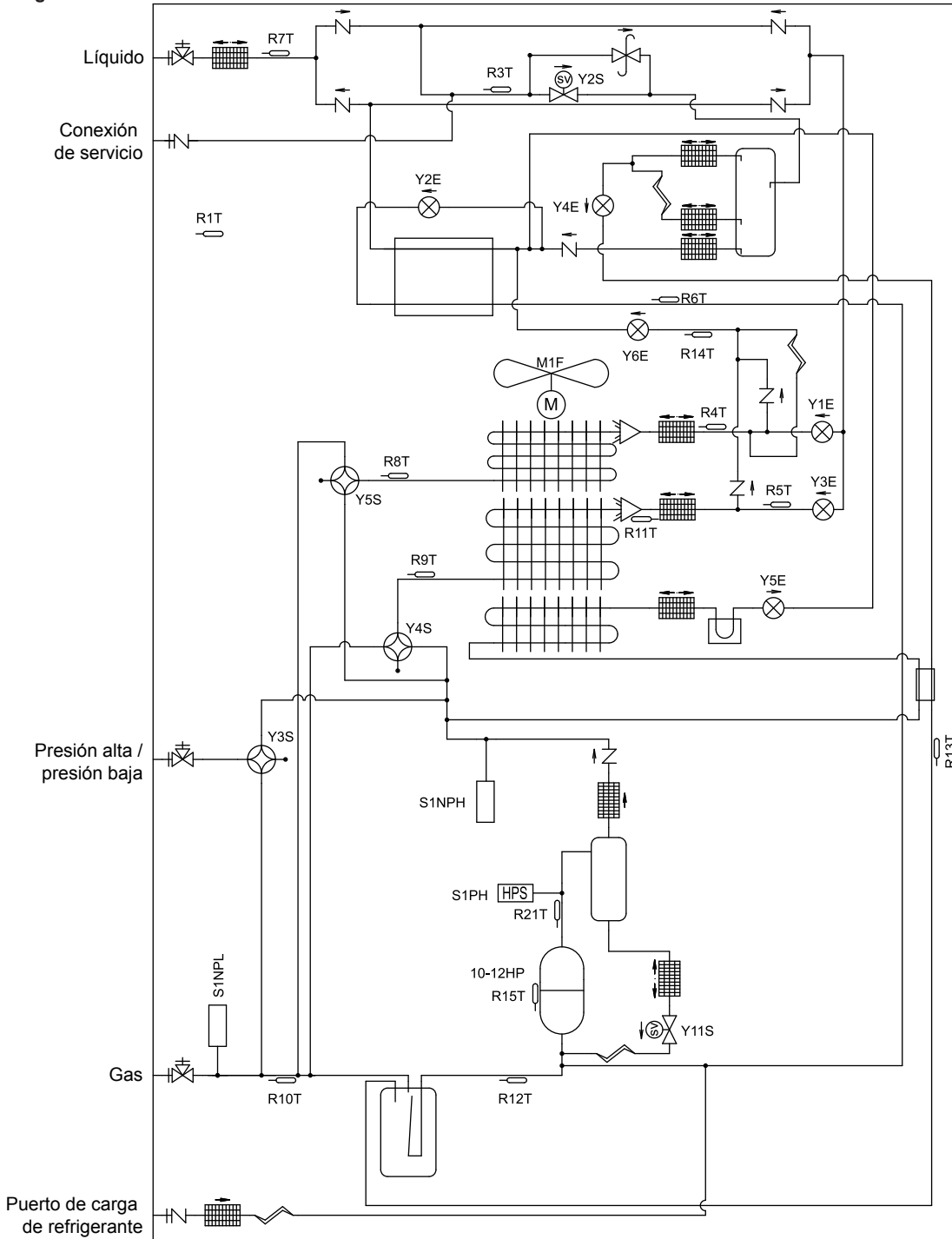
Diagrama de tubería: 5~12 HP
