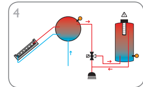
Sistema de termosifón con 2 funciones de termostato (página 12)
