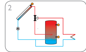
Sistema de energía solar con 1 acumulador y disipación del exceso de calor (página 10)
