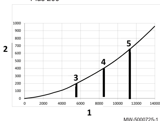
Fig.19 Caídas de presión para POWER HT Plus 200
