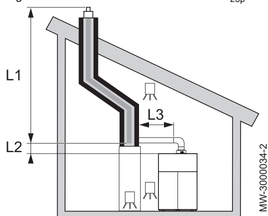
Fig.72 Conductos de humos rígidos B 23p
