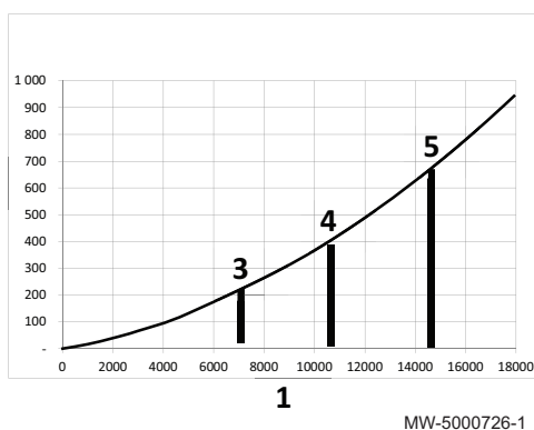
Fig.20 Caídas de presión para POWER HT Plus 250
