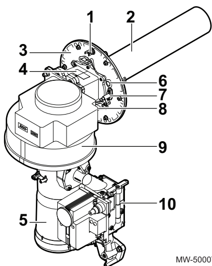
Fig.14 Quemador para POWER HT Plus 200 y POWER HT Plus 250
