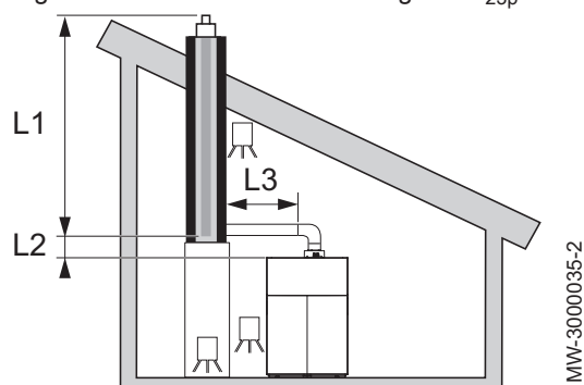
Fig.72 Conductos de humos rígidos B 23p
