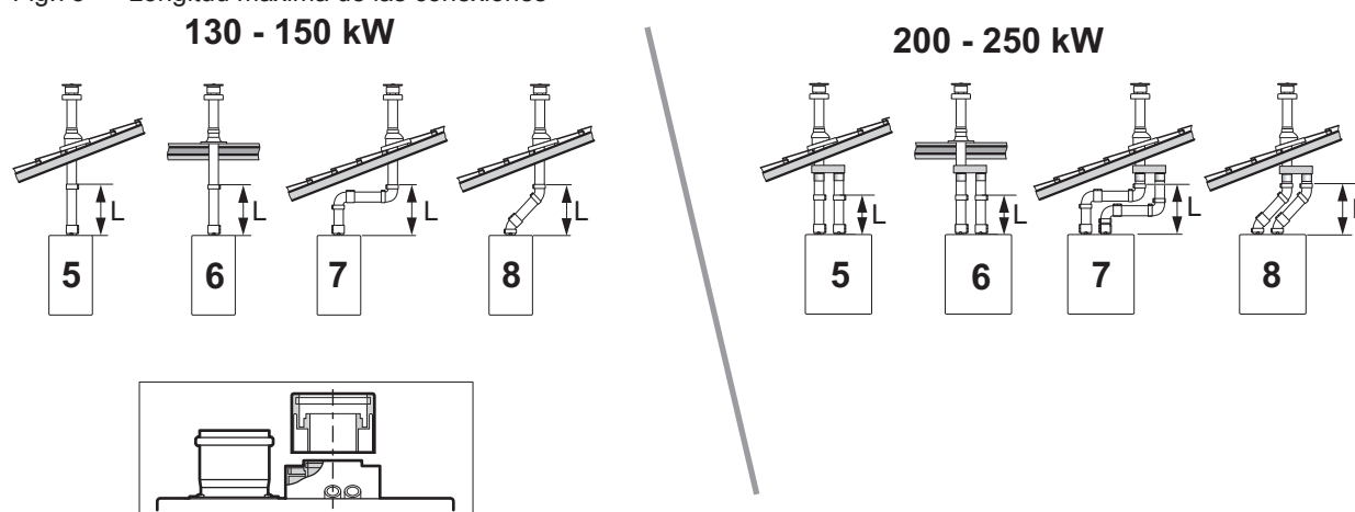
Fig.75 Longitud máxima de las conexiones
