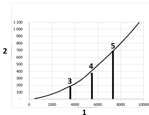
Fig.17 Caídas de presión para POWER HT Plus 130
