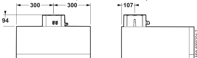
Fig.41 Especificaciones de los conductos coaxiales para POWER HT Plus 90 y POWER HT Plus 110
