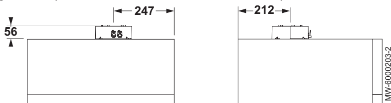
Fig.40 Especificaciones de los conductos coaxiales para POWER HT Plus 50 y POWER HT Plus 70
