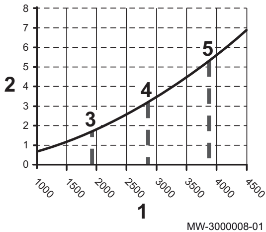
Fig.16 Caídas de presión para POWER HT Plus 70
