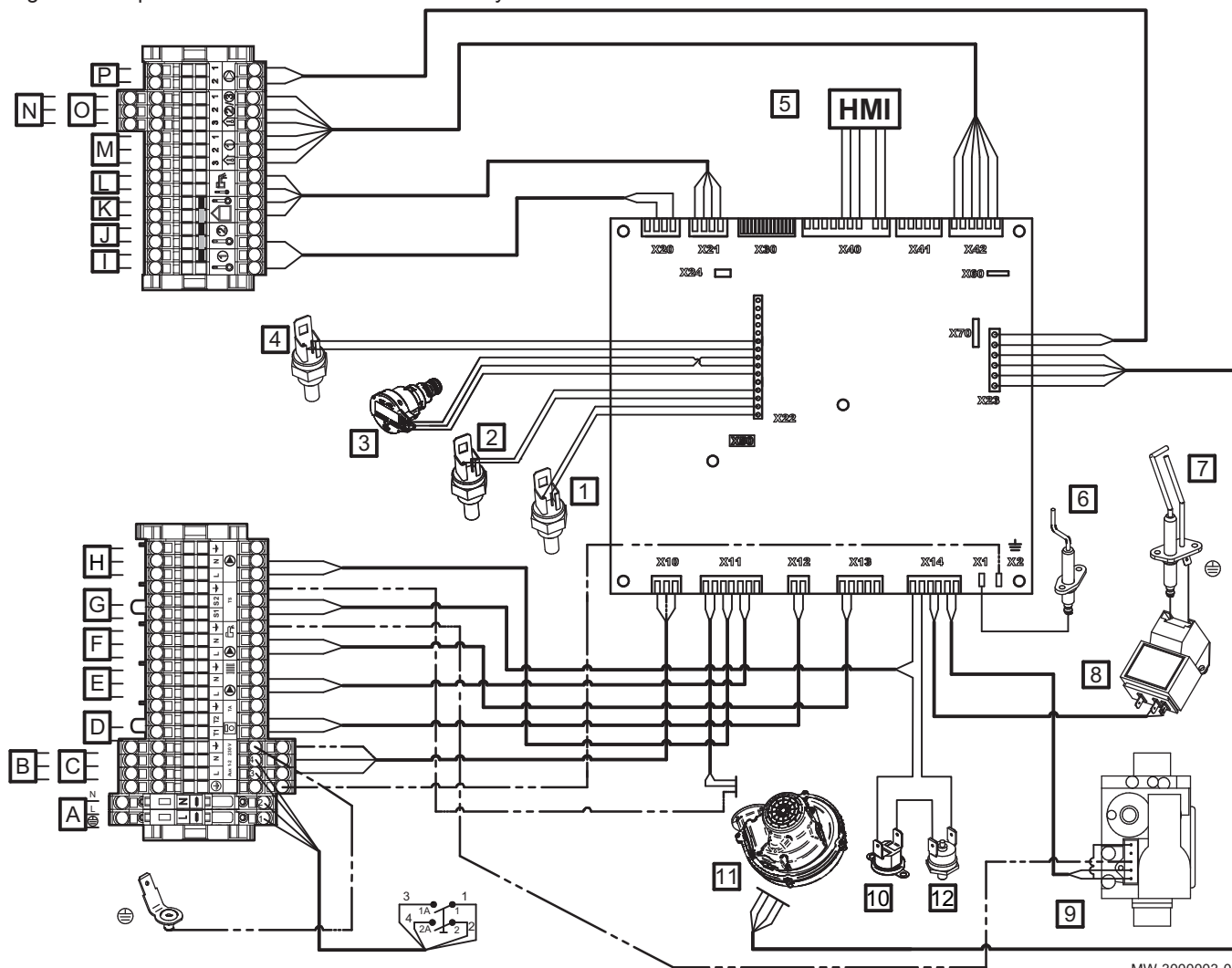
Fig.4 Esquema eléctrico POWER HT Plus 50 y POWER HT Plus 70
