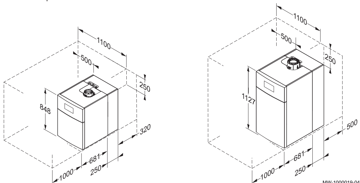
Fig.21 Espacio necesario para las calderas equipadas con un kit de distribuidor sin presión, un kit de intercambiador de calor de placas o un kit de cascada
