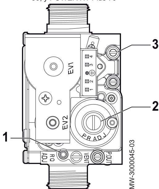
Fig.58 Válvula de gas de POWER HT Plus 90, y POWER HT Plus 110
