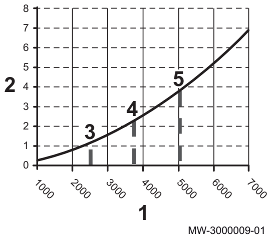
Fig.17 Caídas de presión para POWER HT Plus 90
