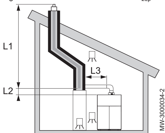
Fig.44 Conductos de humos flexibles B 23p
