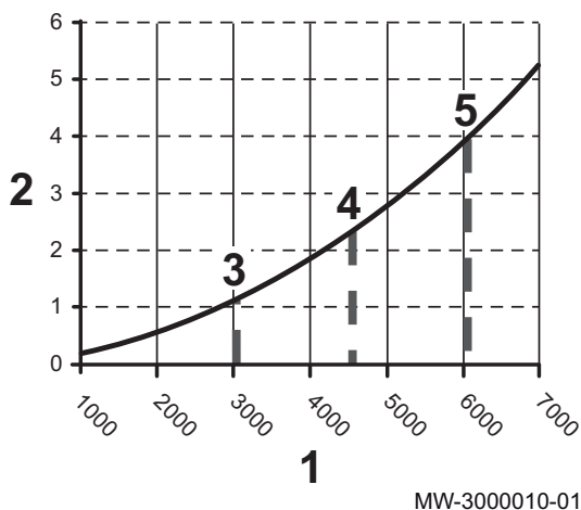
Fig.18 Caídas de presión para POWER HT Plus 110
