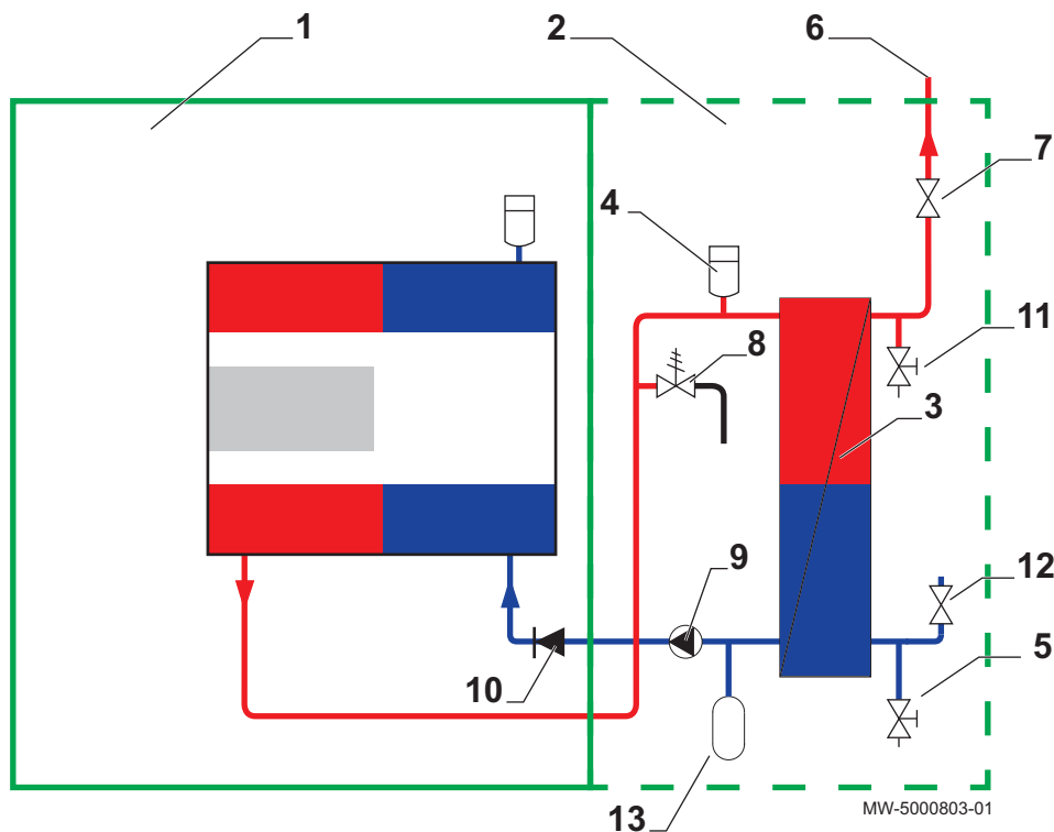
Fig.7 Diagrama funcional de una caldera con intercambiador de calor de placas
