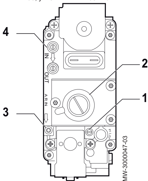
Fig.58 Válvula de gas de POWER HT Plus 90, y POWER HT Plus 110
