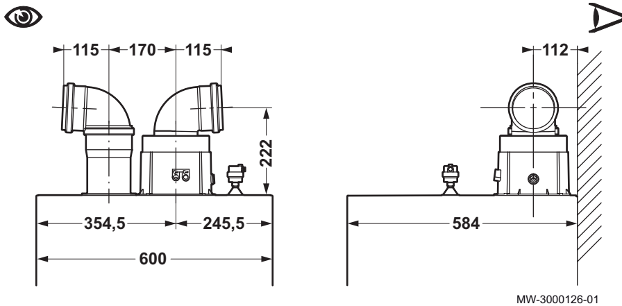
Fig.43 POWER HT Plus 90 y POWER HT Plus 110
