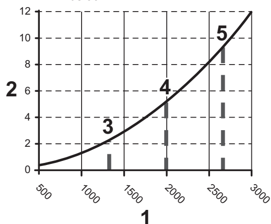
Fig.15 Caídas de presión para POWER HT Plus 50
