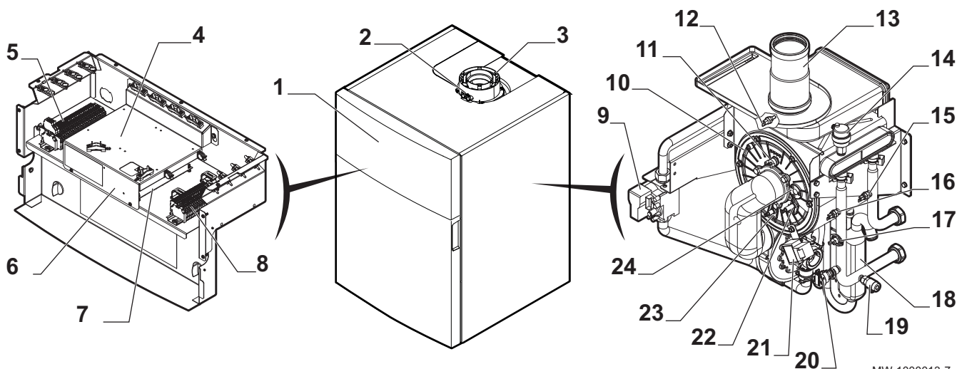
Fig.9 POWER HT Plus 50 y POWER HT Plus 70
