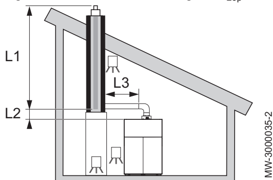
Fig.45 Conductos de humos rígidos B 23p
