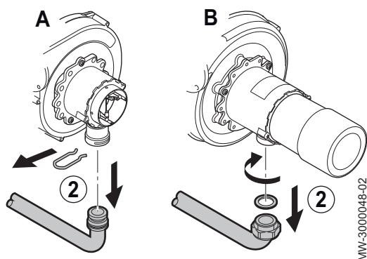
Fig.60 Retirada del venturi
