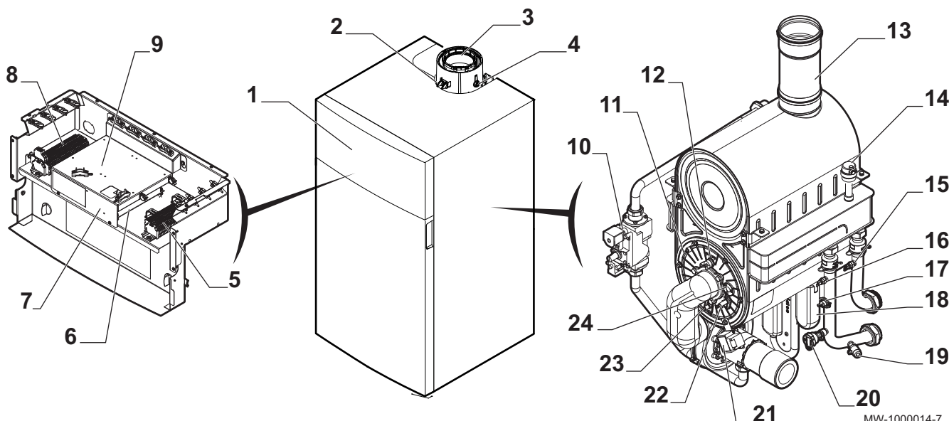
Fig.10 POWER HT Plus 90 y POWER HT Plus 110
