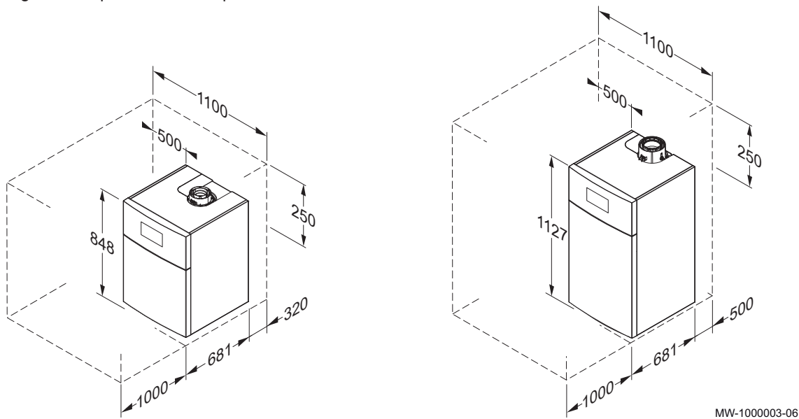
Fig.20 Espacio necesario para las calderas
