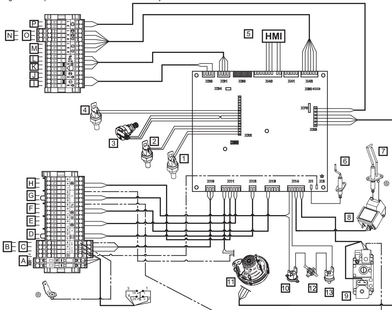
Fig.5 Esquema eléctrico POWER HT Plus 90 y POWER HT Plus 110
