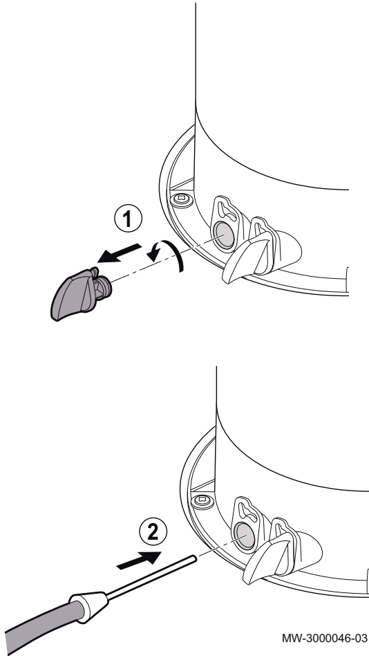
Fig.56 Conexión del analizador de humos
