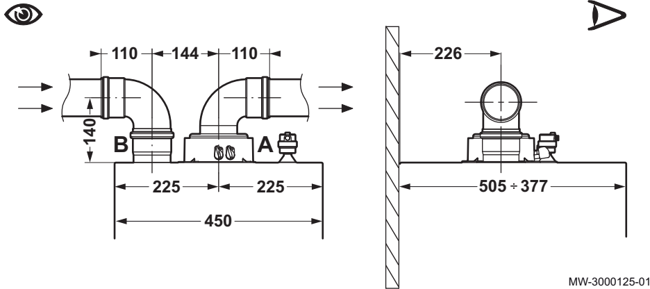
Fig.43 POWER HT Plus 90 y POWER HT Plus 110
