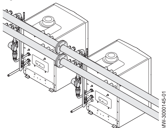
Fig.8 Calderas en cascada
