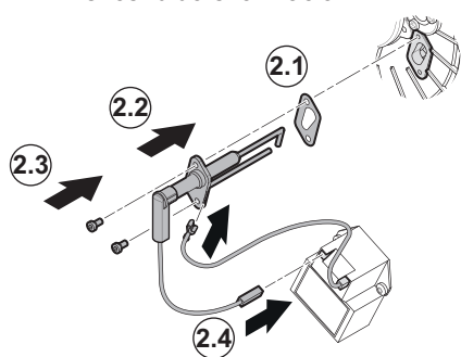
Fig.52 Montaje de los electrodos de encendido e ionización
