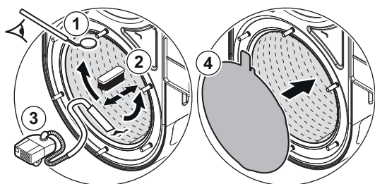
Fig.44 Cepillado y aspiración del intercambiador de calor
