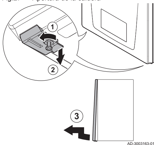
Fig.27 Apertura de la caldera
