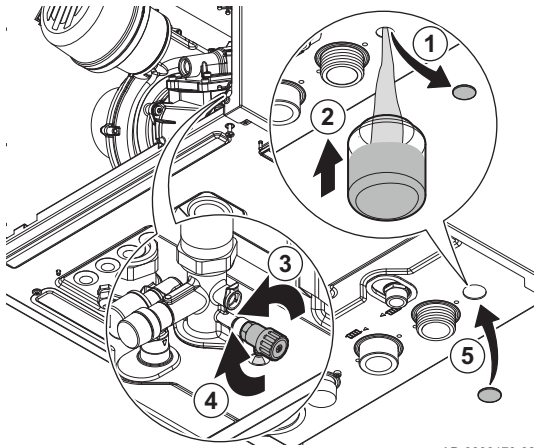
Fig.29 Abrir el grifo de vaciado del intercambiador de calor
