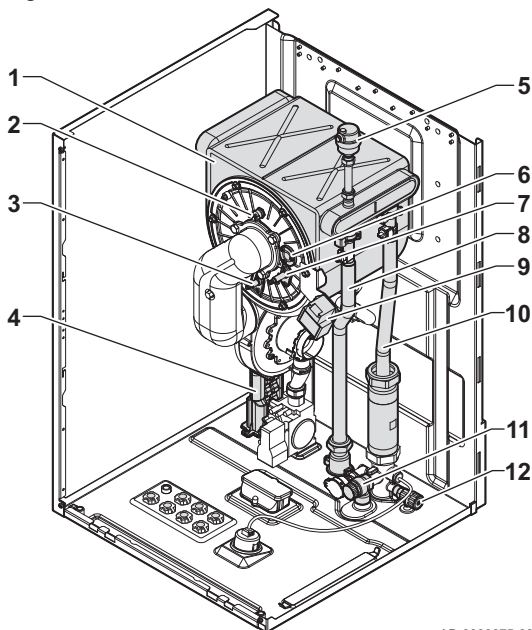
Fig.2 Parte interna
