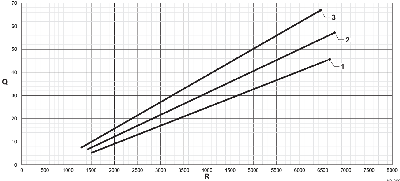
Fig.15 Entrada máxima para calefacción central
