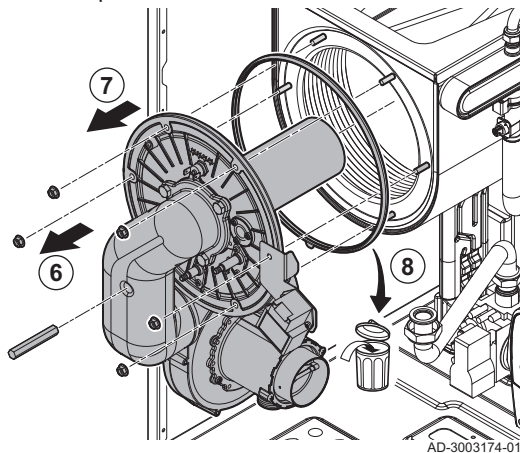
Fig.36 Desmontaje de la unidad de la placa frontal
