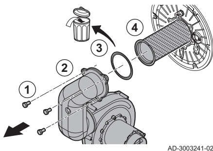
Fig.42 Extracción del quemador en las calderas de los tipos 35 F - 50 F - 70 F.
