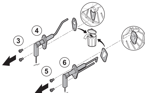
Fig.39 Retirada de los electrodos
