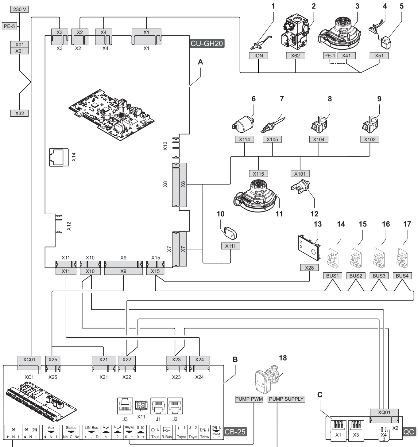
Fig.56 Esquema eléctrico para los tipos de calderas 35 F - 50 F - 70 F
