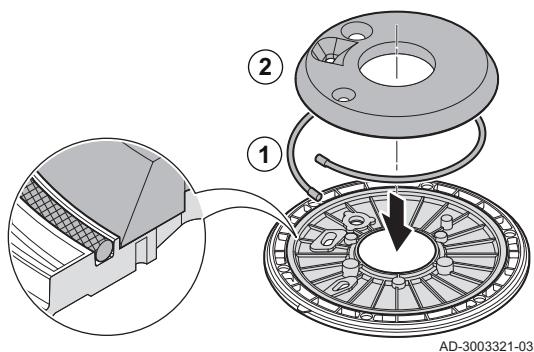
Fig.46 Colocación del aislamiento del quemador y de la junta de cordón de fibra de vidrio
