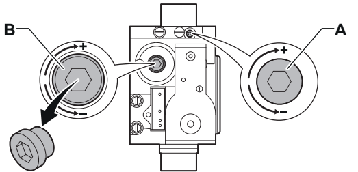
Fig.26 Válvula de control de gas en tipos de caldera:35 F - 50 F - 70 F
