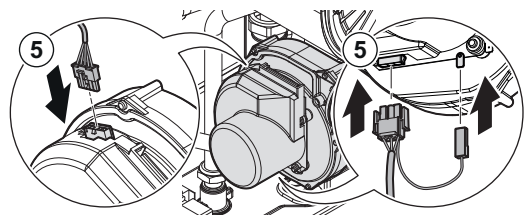
Fig.50 Montaje de los conectores eléctricos del ventilador
