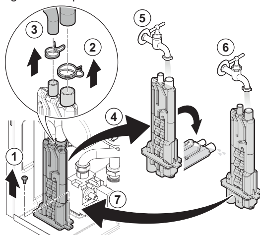
Fig.30 Limpieza del sifón
