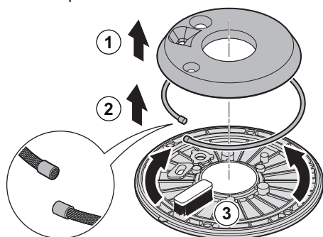
Fig.43 Desmontaje del aislamiento del quemador
