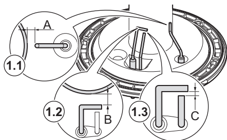
Fig.37 Comprobación de las distancias de los electrodos
