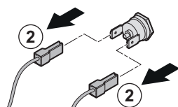
Fig.33 Retirada del cable de ionización
