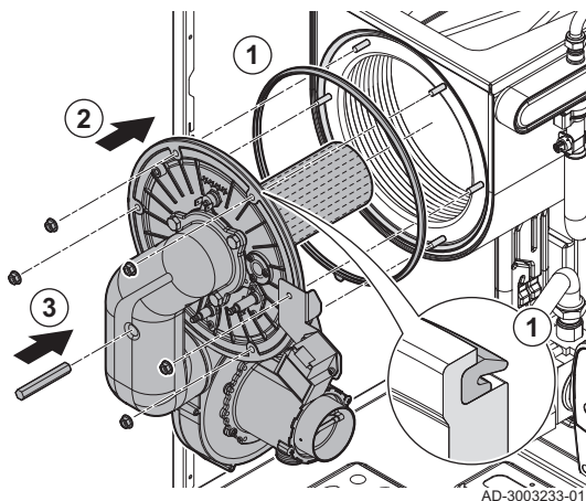
Fig.48 Montaje de la unidad de la placa frontal
