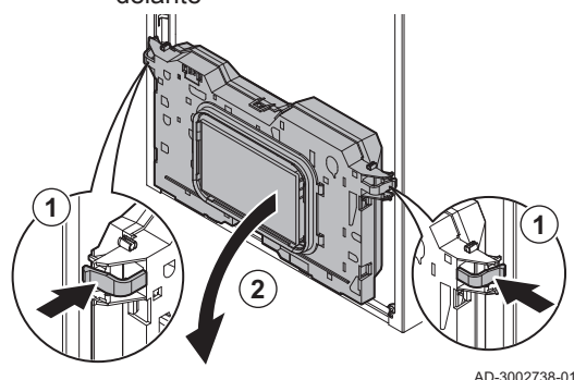
Fig.28 Inclinarse la caja de mando hacia delante
