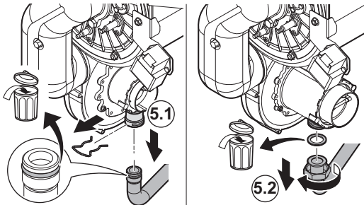
Fig.35 Desmontaje del tubo de gas del tubo de Venturi
