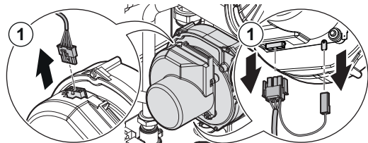
Fig.31 Desmontaje de los conectores eléctricos del ventilador
