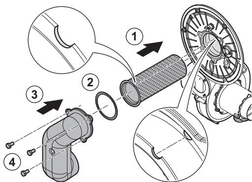
Fig.47 Montaje del quemador en las calderas de los tipos 35 F - 50 F - 70 F.
