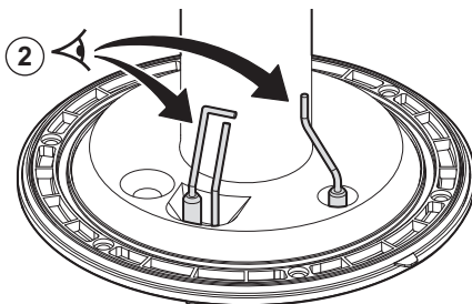
Fig.38 Comprobación del estado de los electrodos de encendido e ionización
