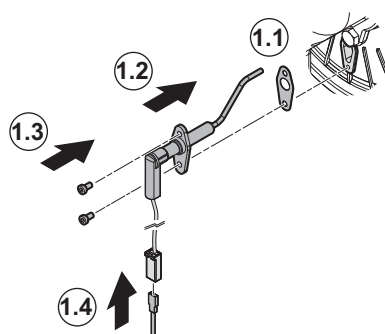
Fig.51 Montaje de los electrodos de encendido e ionización
