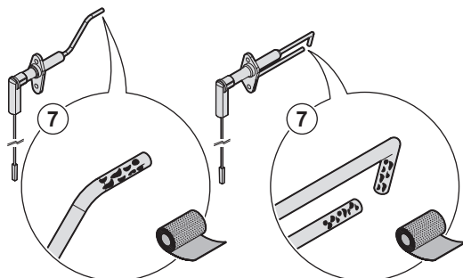
Fig.40 Limpieza de los electrodos
