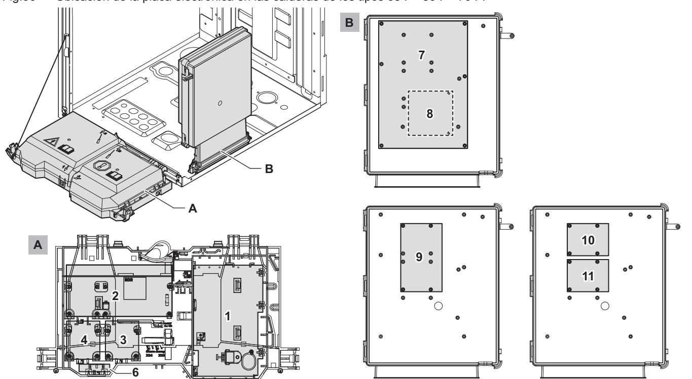
Fig.56 Ubicación de la placa electrónica en las calderas de los tipos 35 F - 50 F - 70 F.
