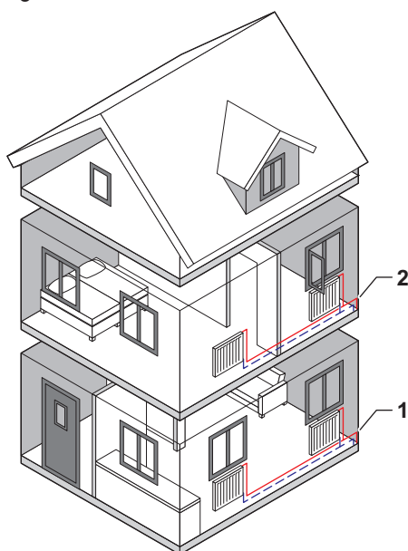
Fig.127 Dos zonas
