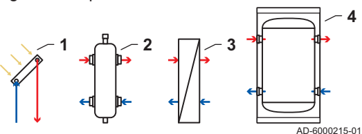
Fig.23 Separación hidráulica
