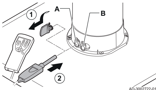
Fig.111 Punto de medición de los gases de combustión y punto de medición de la entrada de aire
