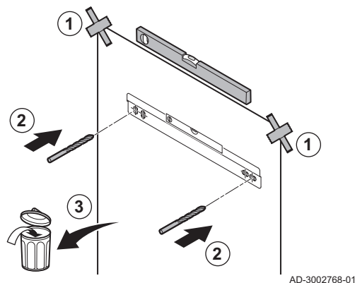
Fig.35 Montaje de la caldera
