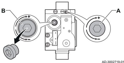
Fig.112 Válvula de control de gas en tipos de caldera:35 F - 50 F - 70 F
