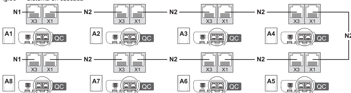
Fig.50 Sistema en cascada
