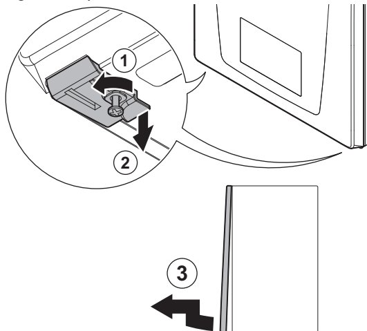
Fig.51 Apertura de la caldera
