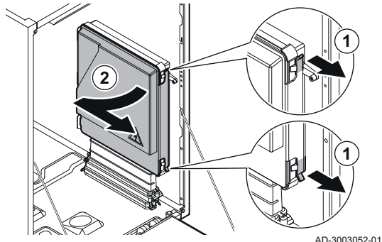
Fig.57 Acceso a la caja de expansión en las calderas de los tipos 35 F - 50 F - 70 F.
