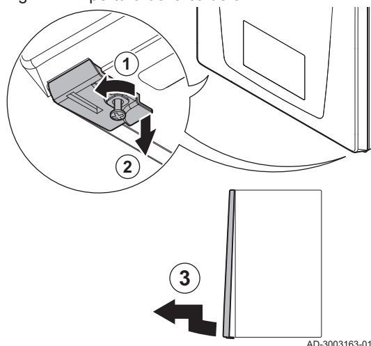
Fig.121 Apertura de la caldera
