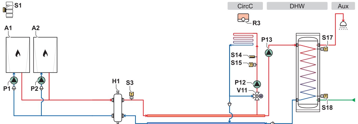
Fig.27 Diagrama y componentes - 6000226
