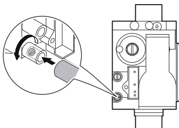
Fig.104 Válvula de control de gas 35 F - 50 F - 70 F
