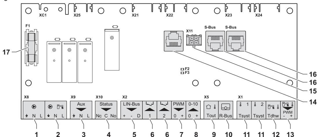
Fig.60 Placa electrónica de conexión CB-25
