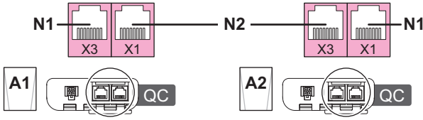
Fig.30 Conexiones S-bus
