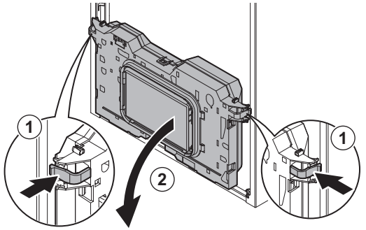
Fig.52 Inclinar la caja de mando hacia delante
