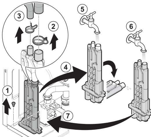
Fig.124 Limpieza del sifón
