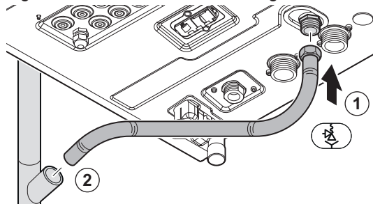
Fig.43 Conectar la válvula de seguridad
