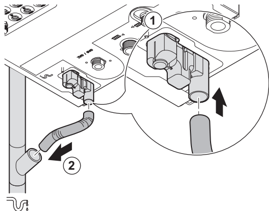
Fig.42 Conexión del tubo de desagüe de condensados
