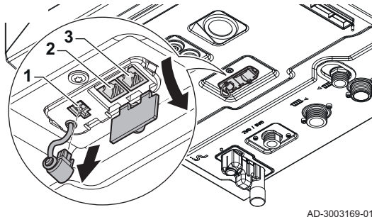
Fig.47 Ubicación del conector Quick connect
