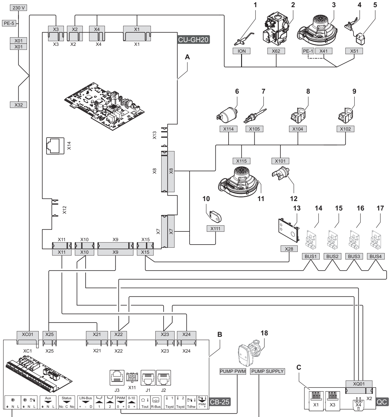
Fig.149 Esquema eléctrico para los tipos de calderas 35 F - 50 F - 70 F
