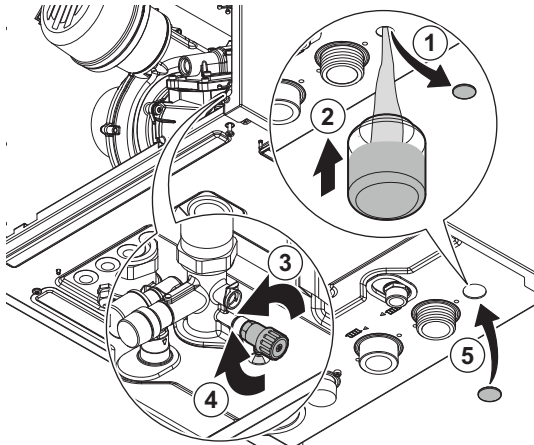
Fig.123 Abrir el grifo de vaciado del intercambiador de calor
