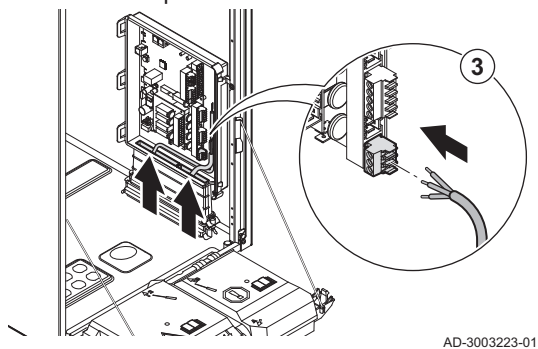
Fig.59 Tendido de cables dentro de la caja de expansión para las calderas de los tipos 35 F - 50 F - 70 F
