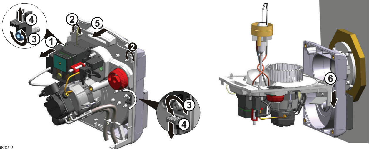
Fig.76 Colocación del quemador en posición
