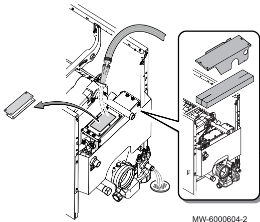
Fig.75 Limpieza del cuerpo del condensador
