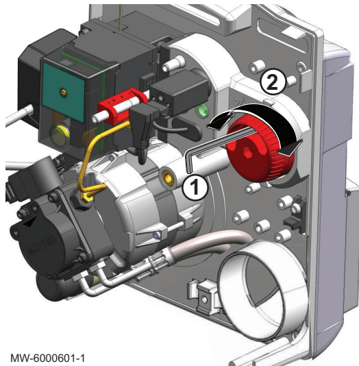
Fig.47 Ajuste de la compuerta de aire
