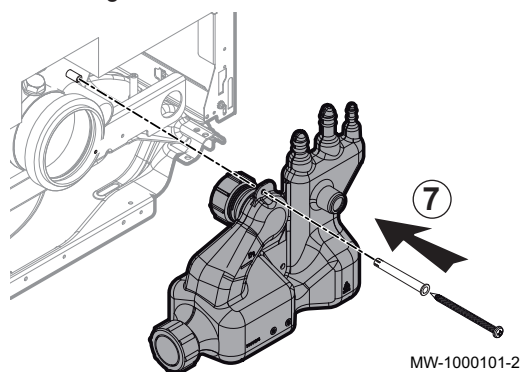
Fig.38 Colocar de nuevo el sifón en su lugar
