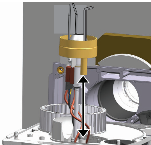
Fig.78 Control de la célula de detección de llama
