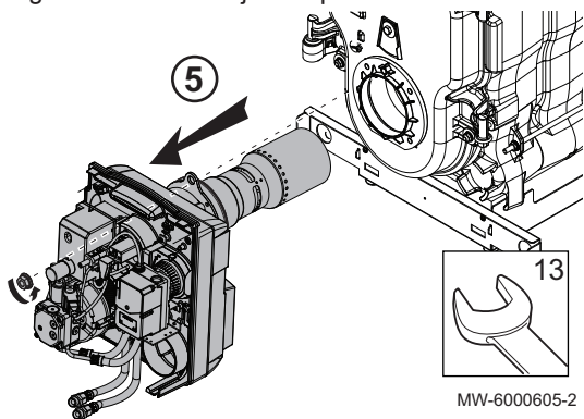
Fig.72 Desmontaje del quemador
