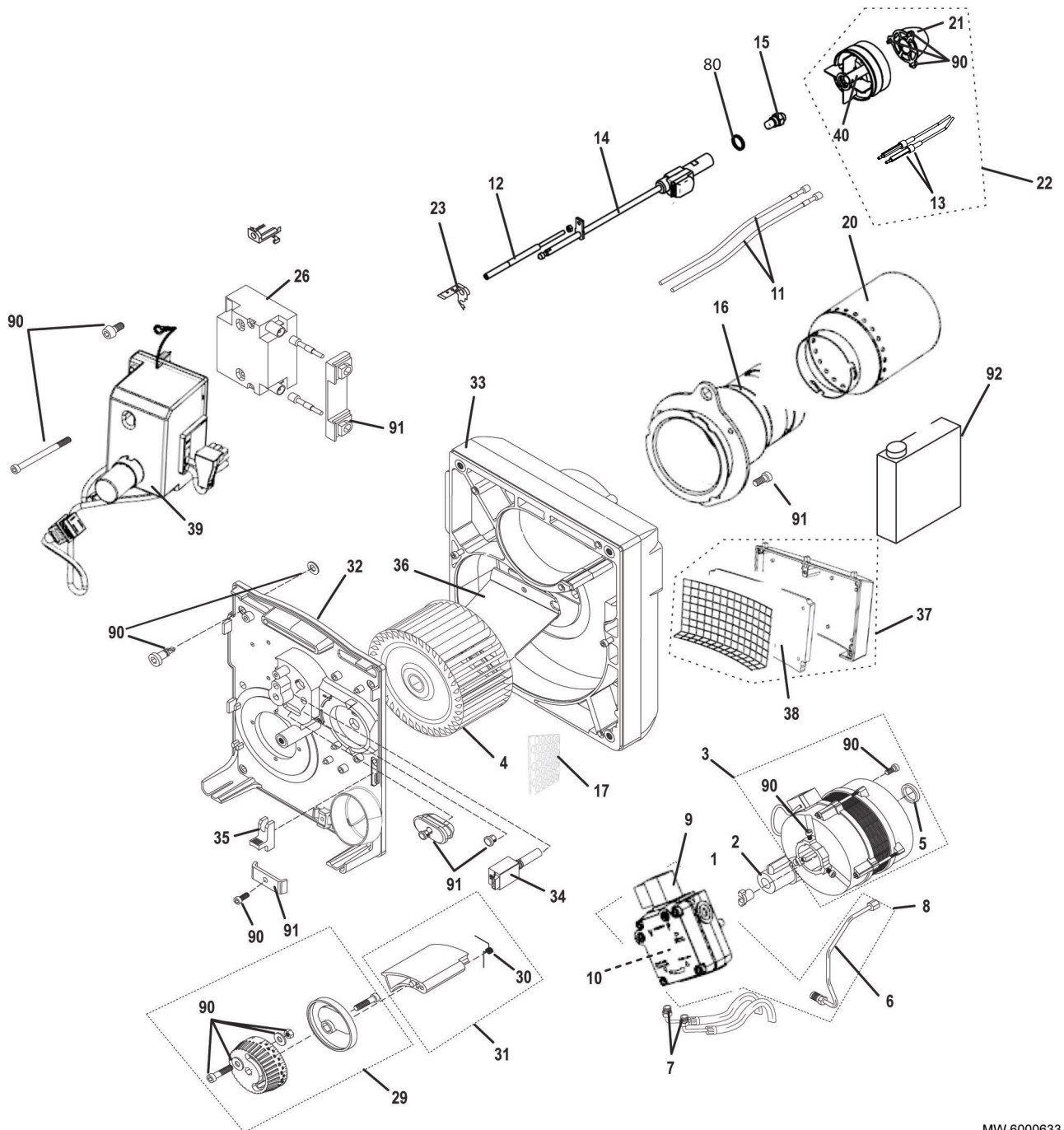
Fig.92 Quemador
