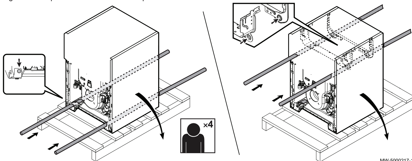
Fig.12 Manipulación con barras de transporte
