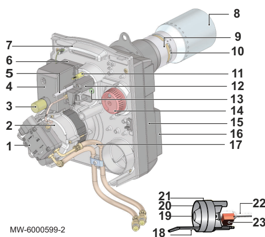
Fig.5 Componentes principales
