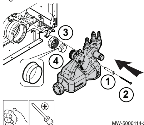
Fig.14 Colocación del sifón
