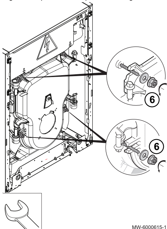
Fig.74 Limpieza del cuerpo de la caldera
