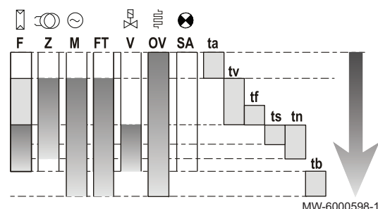
Fig.6 Esquema de funcionamiento
