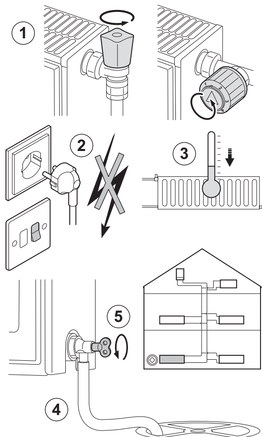
Fig.81 Vaciado de la instalación
