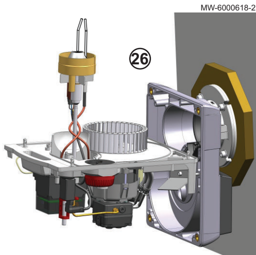
Fig.79 Limpieza del ventilador
