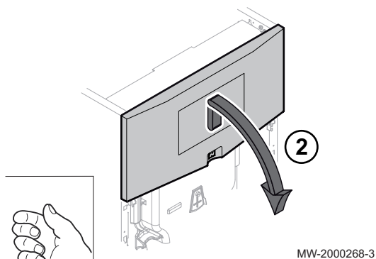
Fig.69 Retirada el panel frontal superior
