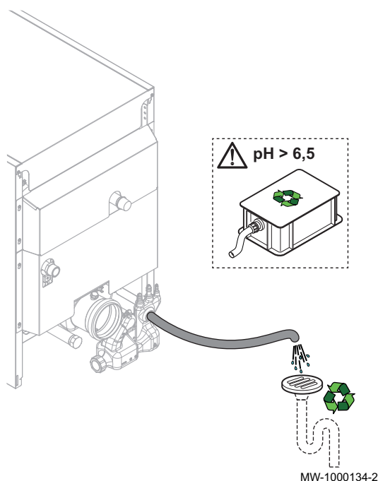
Fig.15 Conexión del conducto de evacuación de los condensados
