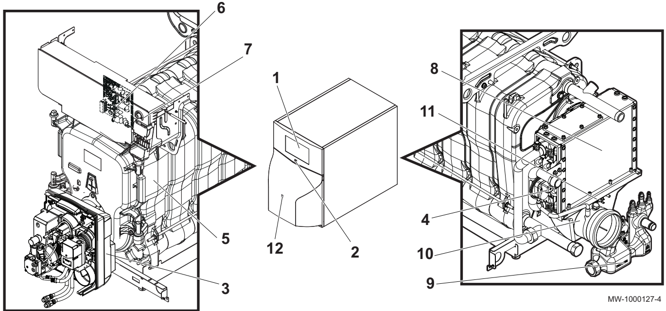
Fig.4 Componentes principales
