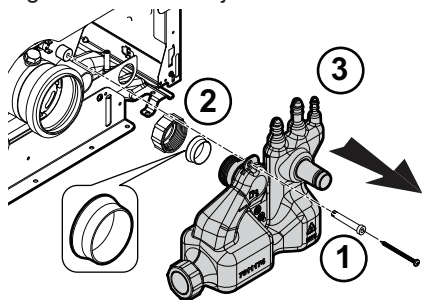
Fig.36 Desmontaje del sifón
