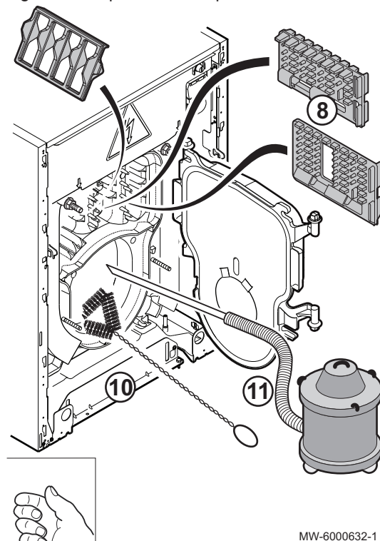
Fig.74 Limpieza del cuerpo de la caldera
