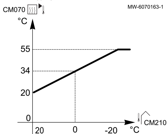
Fig.56 Curva de calefacción sin pie de curva
