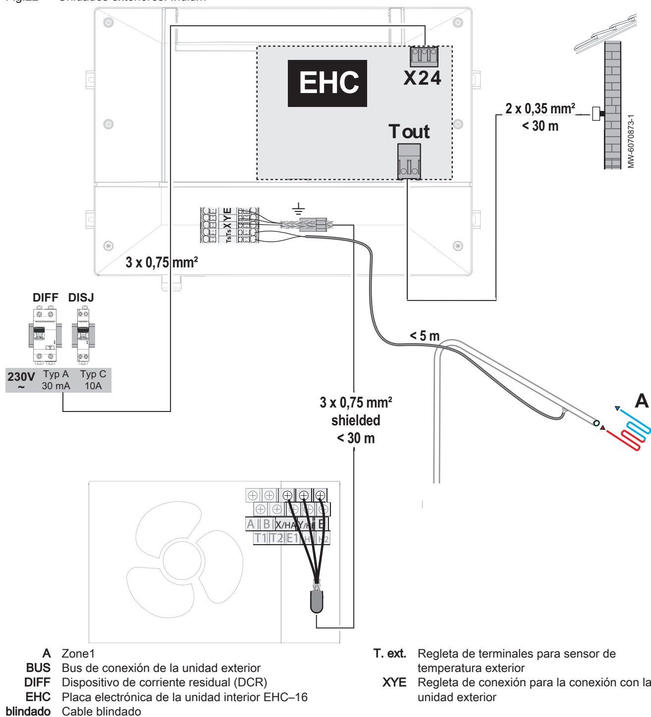
Fig.22 Unidades exteriores: Iridium
