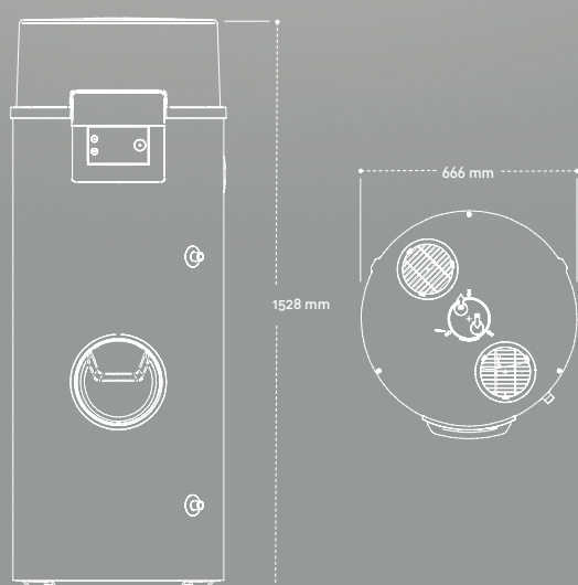
BC ACS IN 200 y BC ACS 1E 200 (mm) Ø200
