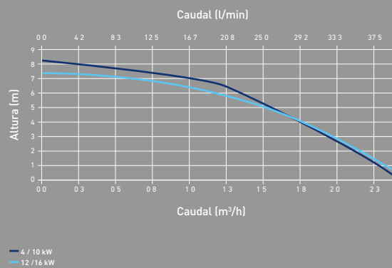
Presión disponible a la salida de la bomba de calor
