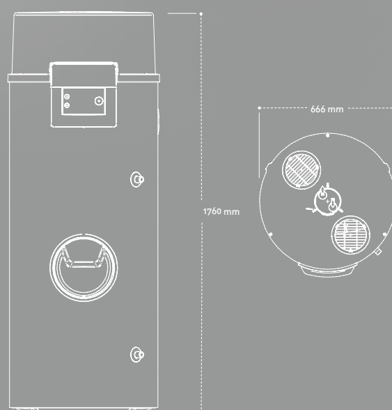
BC ACS IN 300 y BC ACS 1E 300 (mm)
